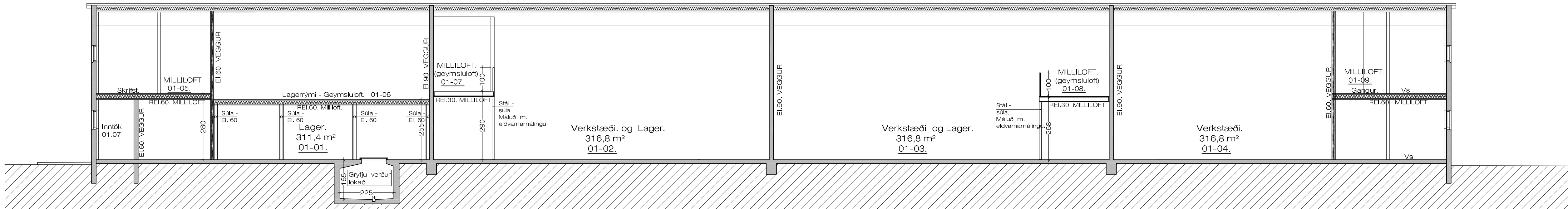
SNID C - C 1:100
